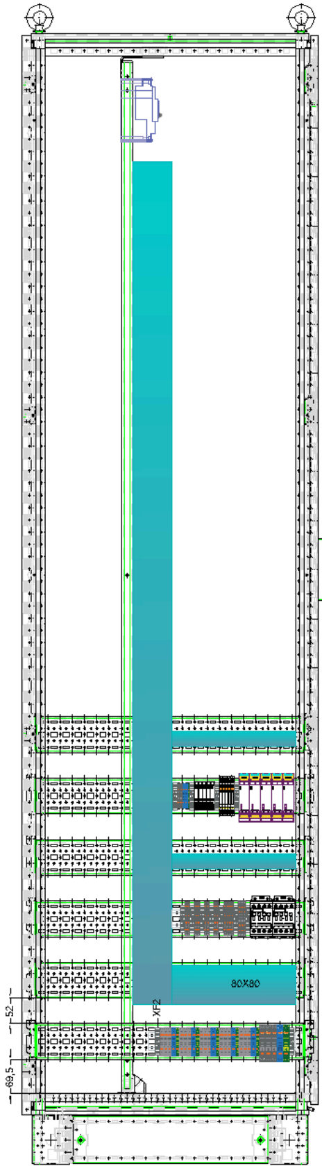
LAYOUT INTERNO - LATERAL
